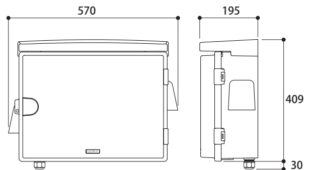
HEA-007W LEDIUSローボルトトランス600W
