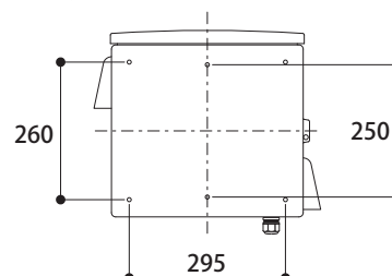
【図④】 本体背面取付面
